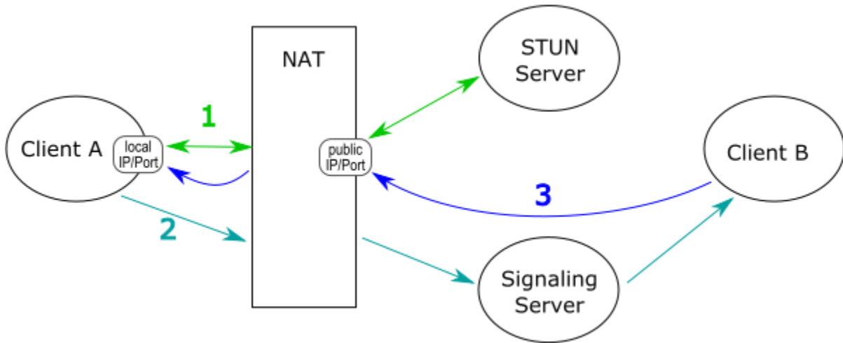
Abb. 3: Erfolgreiche Kommunikation unter Zuhilfenahme eines STUN-Servers.
